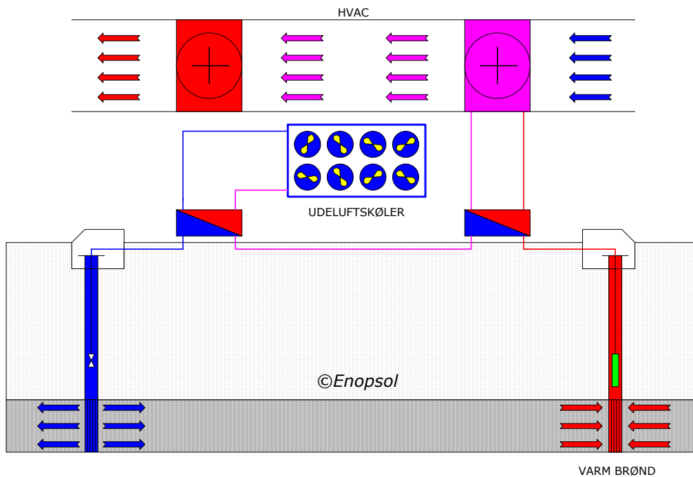
Figur 4. ATES vintertid. For-opvarmning med grundvand og kuldagring med kold udeluft.
